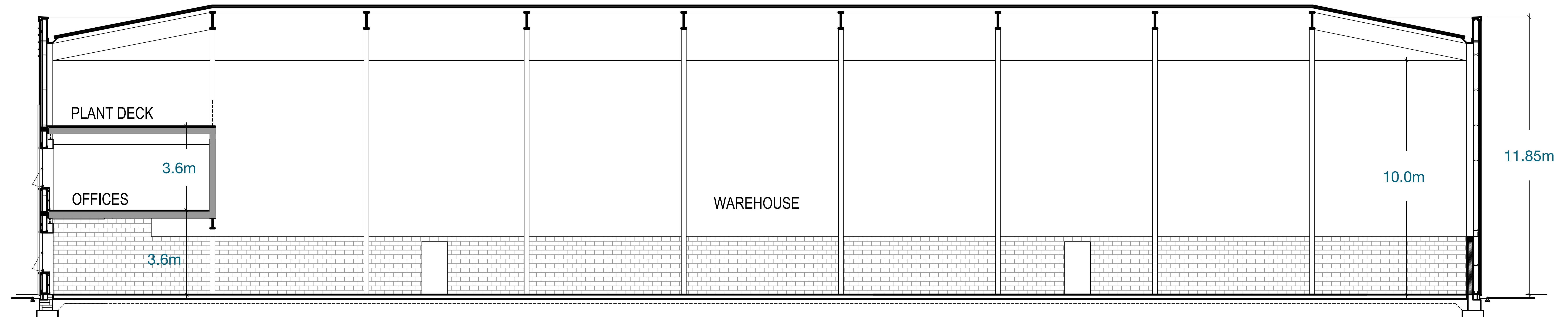
LONGITUDINAL SECTION
